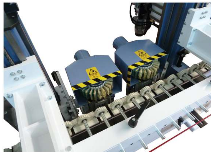
SZLIFOWANIE KRAŻKIEM ŚCIERNYM
