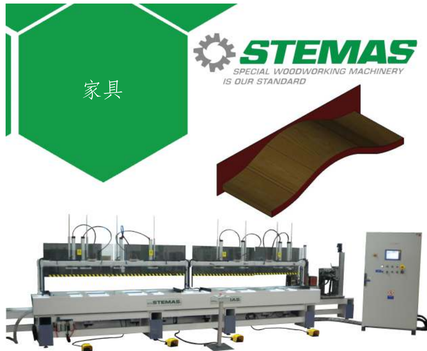
WAVE 是2或4轴数控控制，可加工曲面工件的封边和修边。
